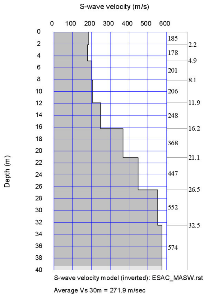
Ricostruzione stratigrafica indicativa congiunta ESAC – MASW
