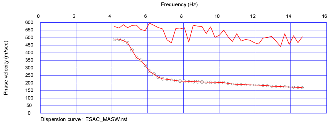
Curva di dispersione congiunta ESAC - MASW
